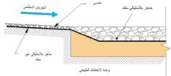
شكل 14. الفرش الركامي المنحدر باتجاه وحدة الاحتفاظ الطبيعي.
