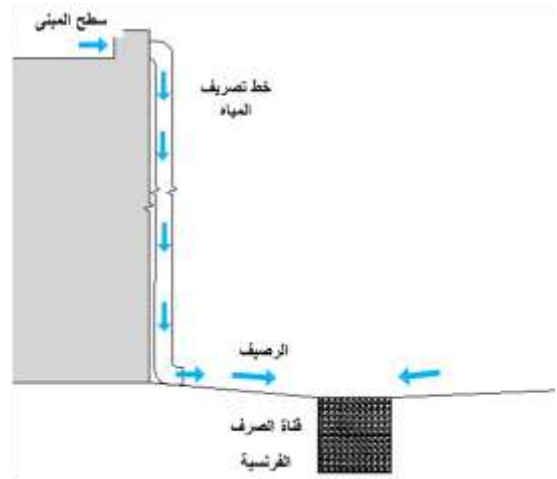
شكل 13. وظائف قناة التصريف الفرنسية.
