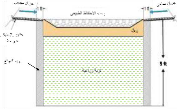
شكل 16 . حدود تخزين المياه في التربة.
