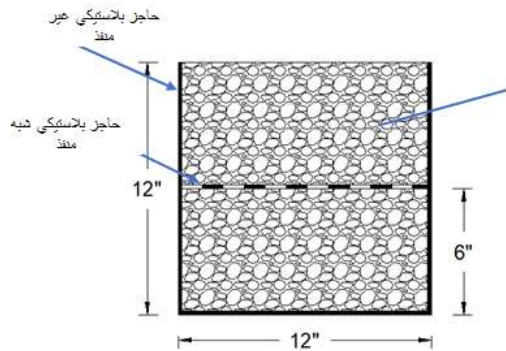
شكل 12 . مقطع عرضي لقناة التصريف الفرنسية.
