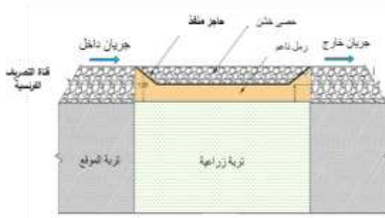
شكل 11 . مقطع عرضي لوحدة الاحتفاظ الطبيعي.
