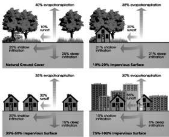
شكل 1. تأثير التطور العمراني على الدورة الهيدرولوجية لمياه الأمطار [1]
