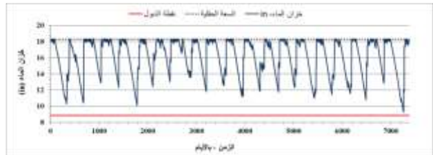
شكل 17 . التغير في المياه المخزنة في حالة مساحة التاج الأخضر معتدلة.
