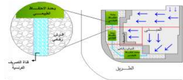
شكل 10 . موقع تقنيات LID ومسار الجريان السطحي.
